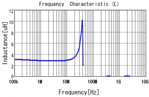
■ 1264EY-3R3N L
